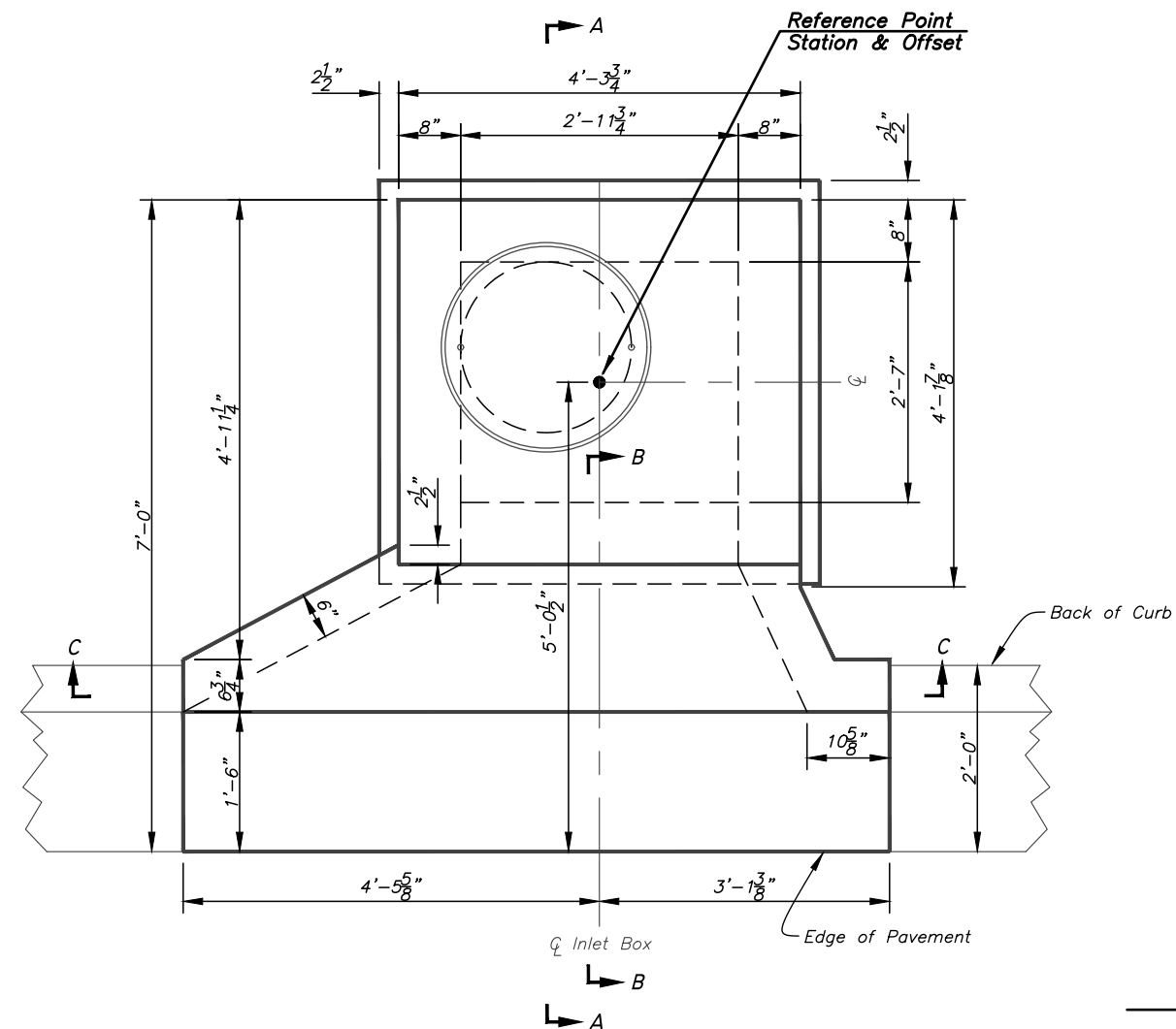
PLAN Scale: 1/2" = 1'-0"
