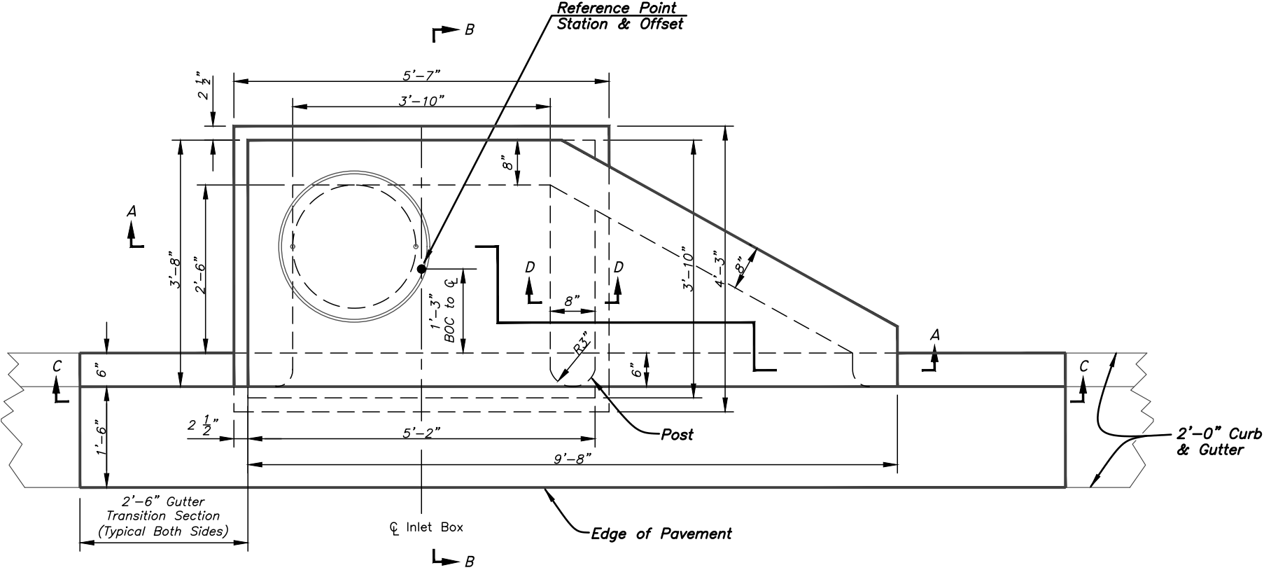
PLAN Scale: 1/2" = 1'-0"
