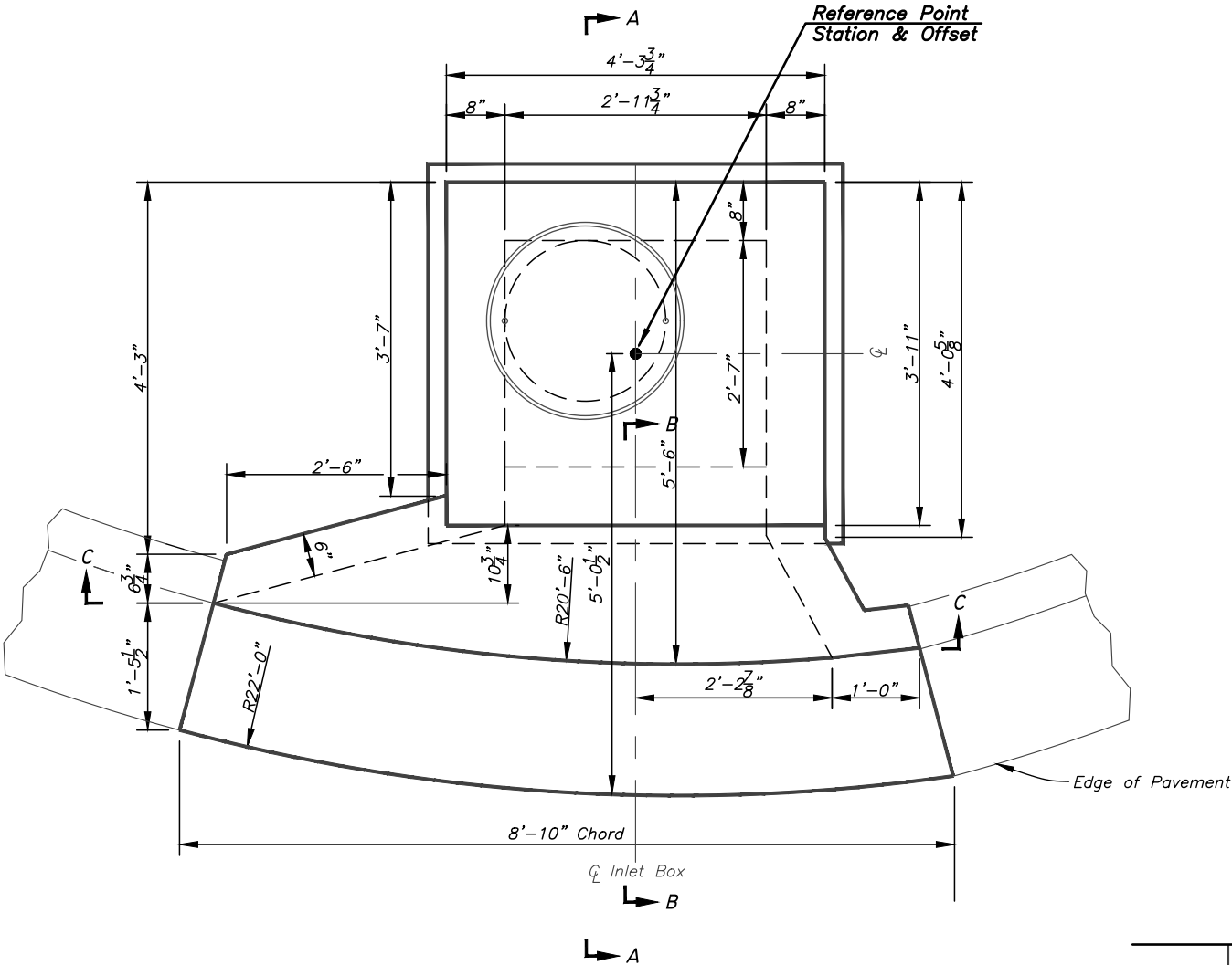
PLAN Scale: 1/2" = 1'-0"
