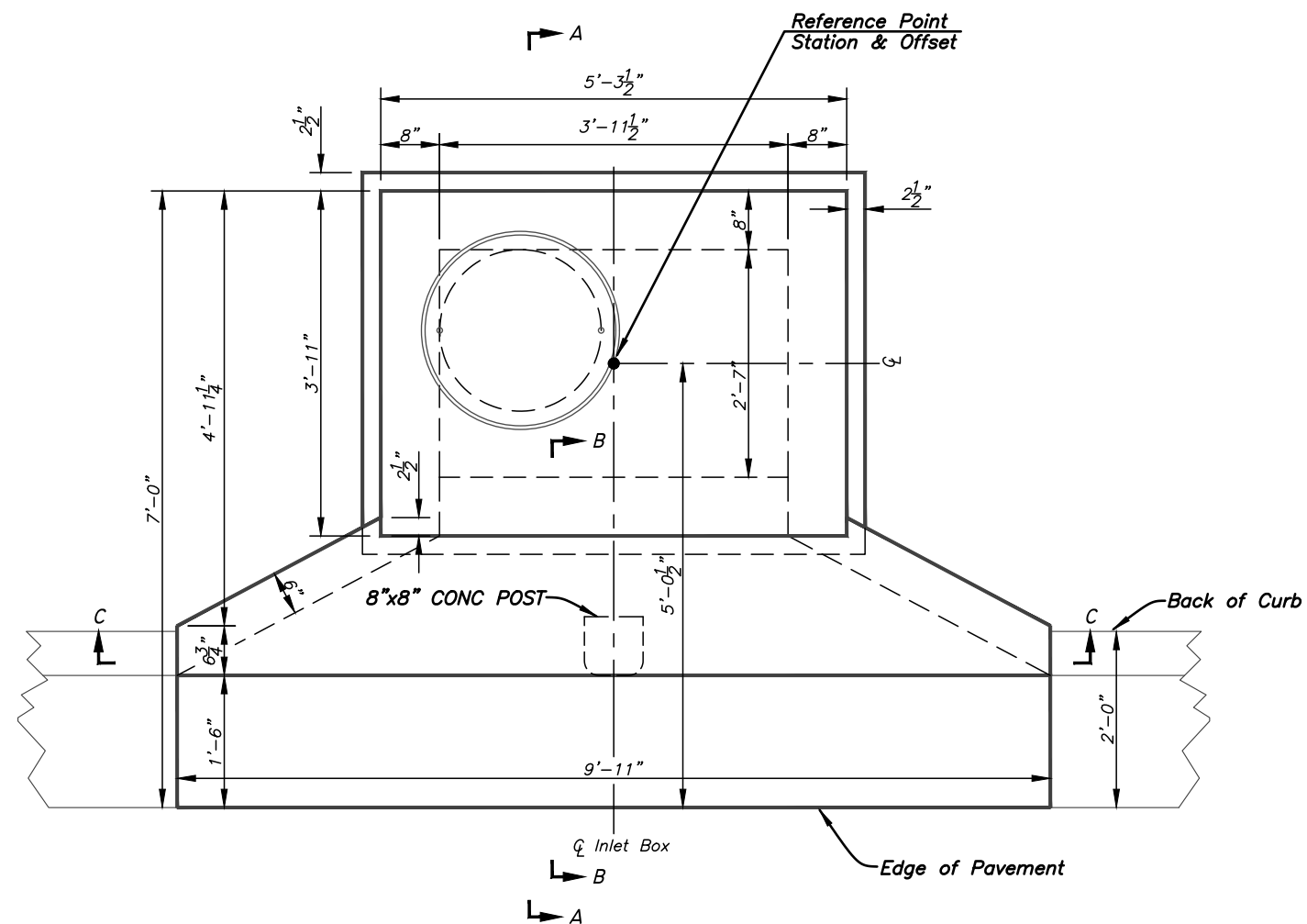
PLAN Scale: 1/2" = 1'-0"
