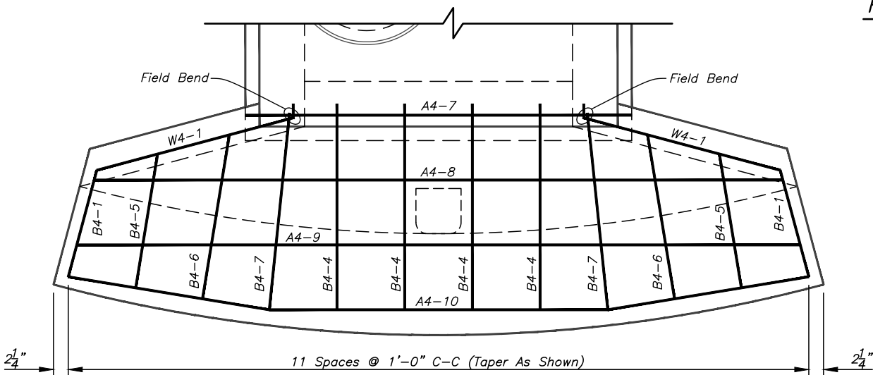
PLAN Scale: 1/2" = 1'-0"
