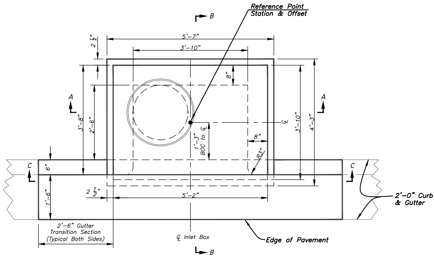
PLAN Scale: 1/2" = 1'-0"
