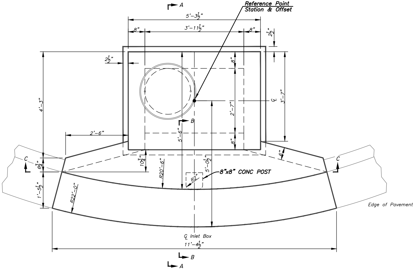
PLAN Scale: 1/2" = 1'-0"
